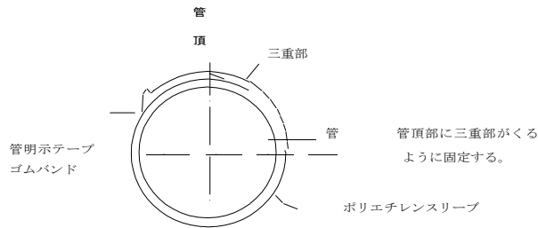
図3.8.1 スリーブの固定方法
