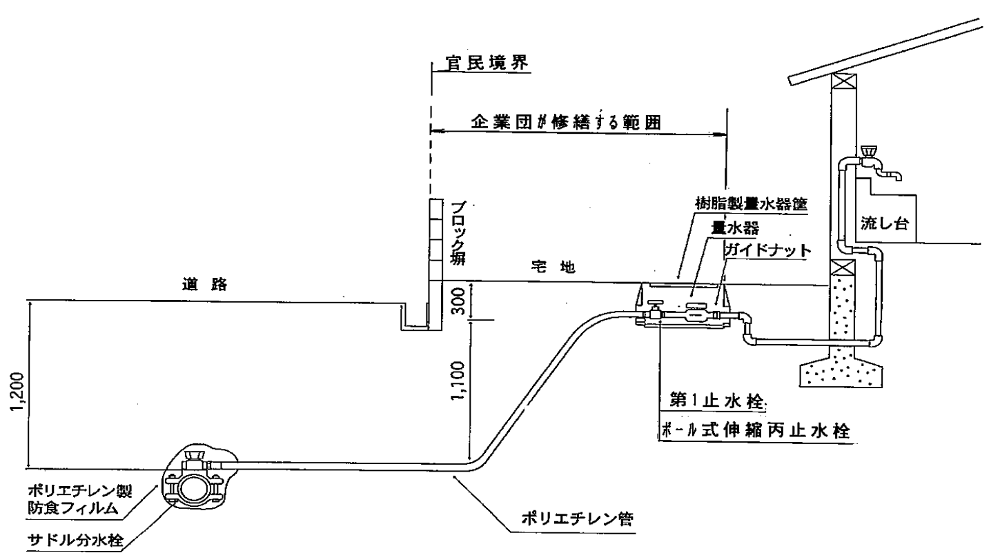
図2.10.1 給水装置標準図
