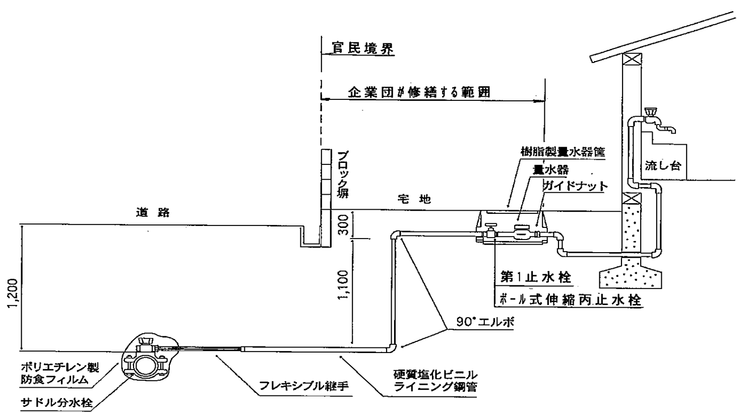
図2.10.2 給水装置標準図
