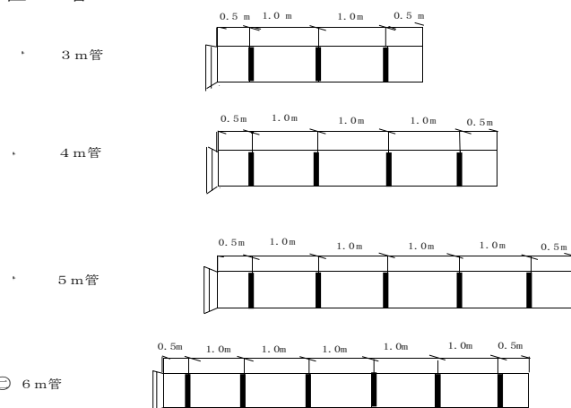
明示テープ貼付標準図
